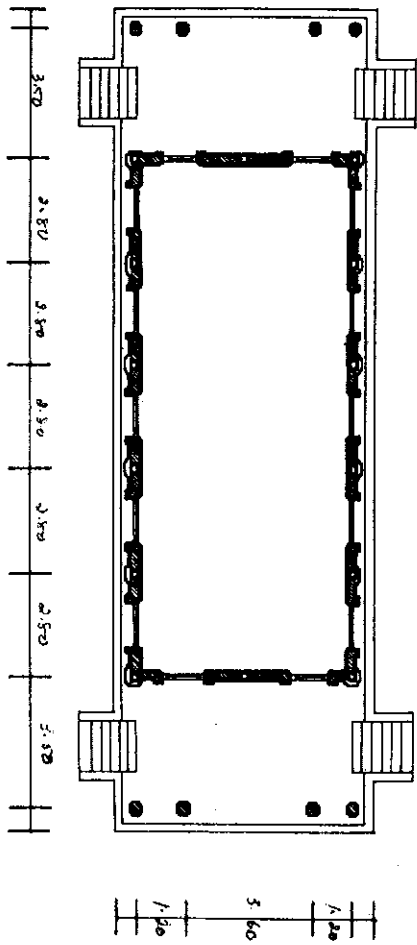
แบบแปลน 1:3,100
