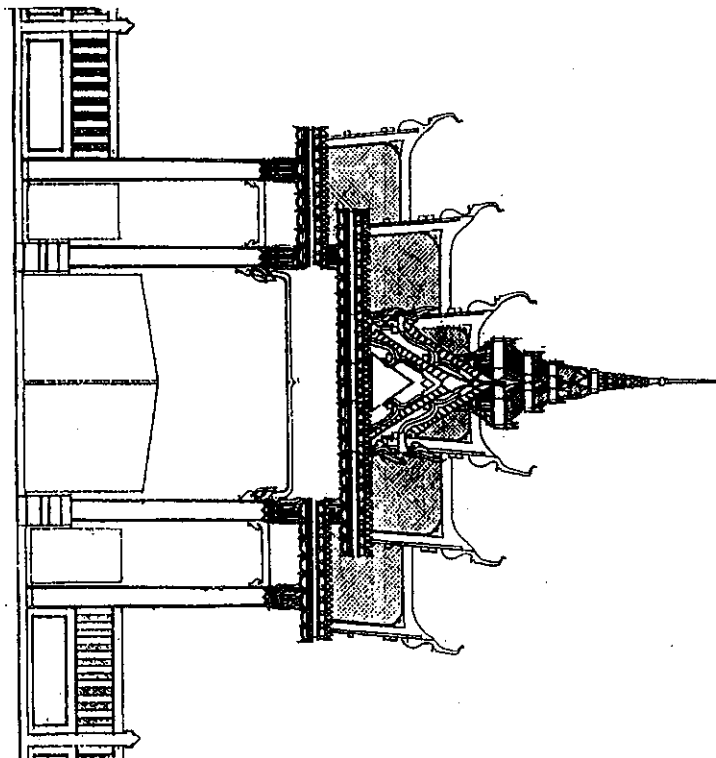
แบบรูปด้านหน้า 1 : 100
