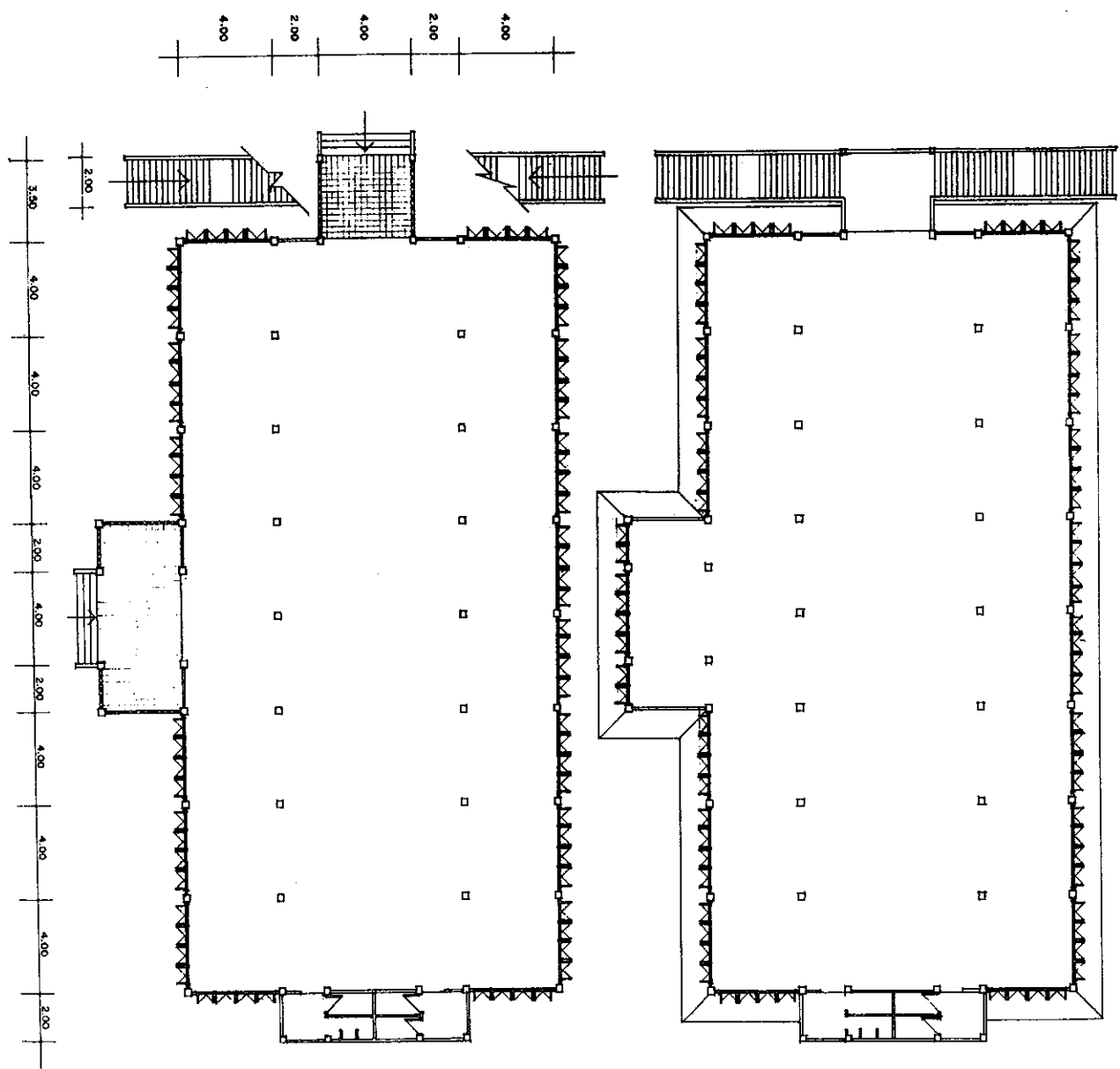
แปลนชั้นล่าง
